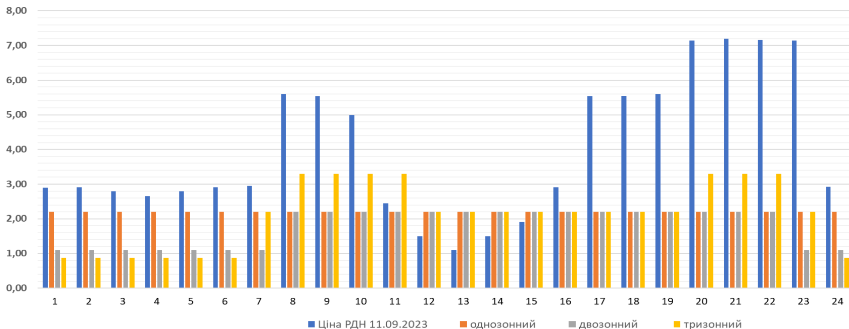
Погодинні ціни на електроенергію, грн/кВт*год, без ПДВ
